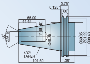
CAT50
