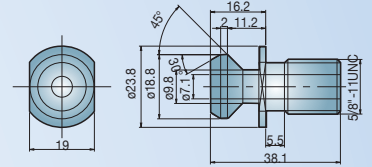
ANSI CAT40
